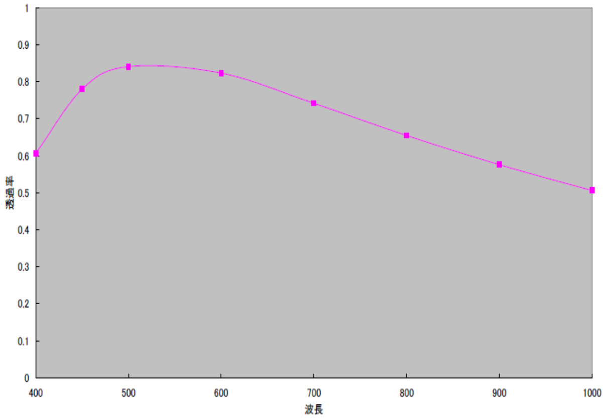
LMVZ4411 (991) 透過率
