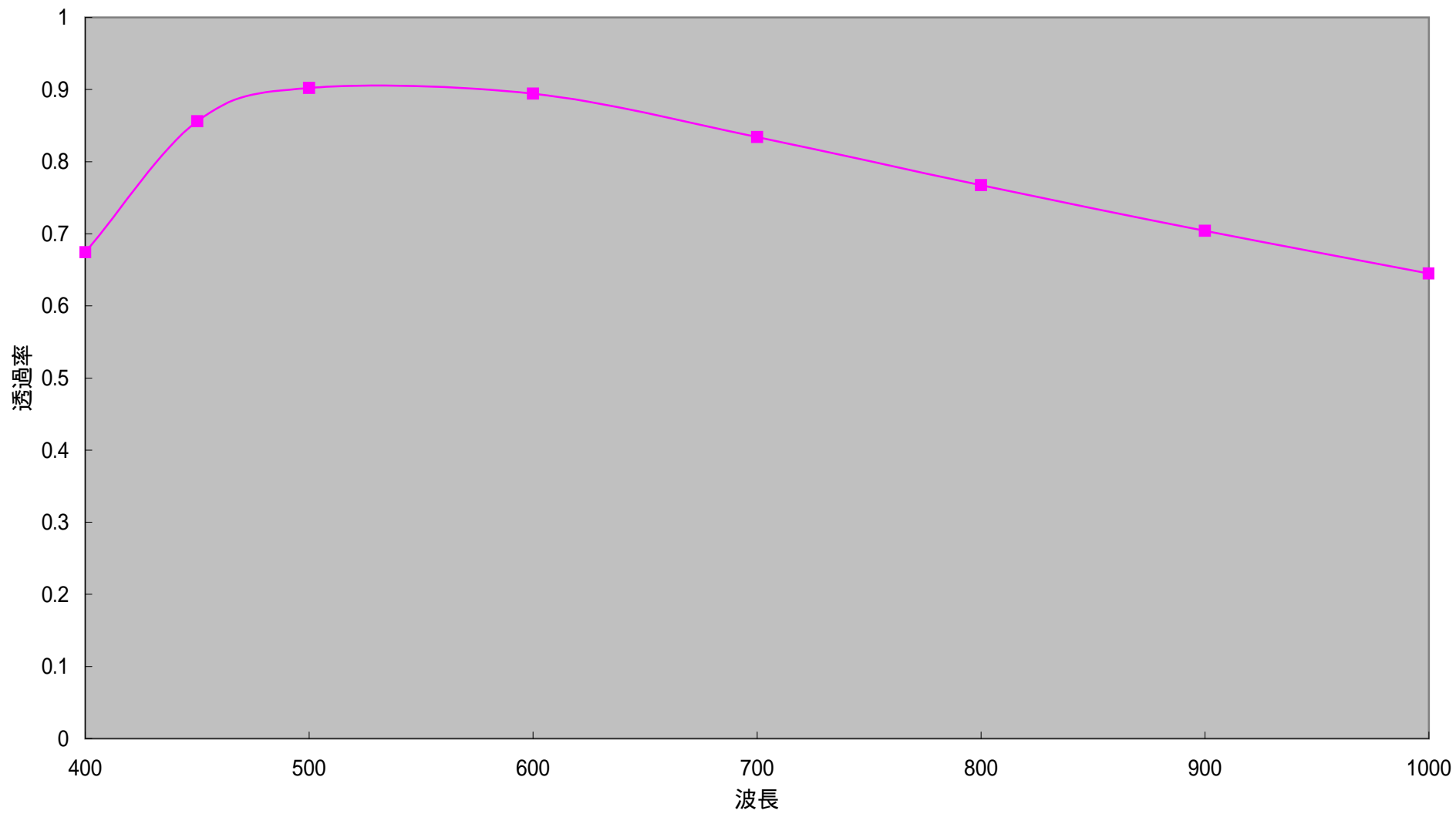
LM8JC (637) 透過率
